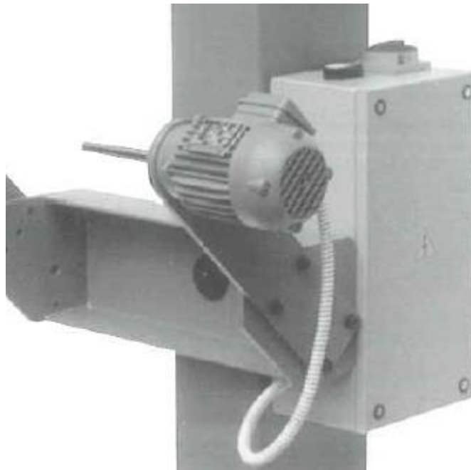
Particolare rullo ribattitore cava:
